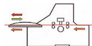
Schemat drogi prowadzenia papieru
